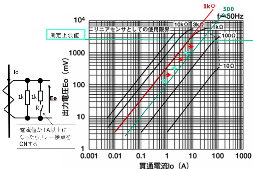
図5 CTセンサによる測定レンジ拡大方法
