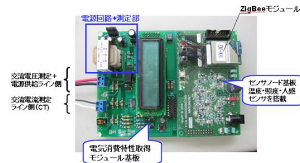
図4 電気消費特性取得モジュールの仕様及び試作モジュール
