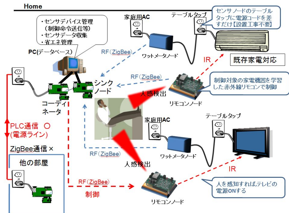
図1 PLC/ZigBee 相互補完通信による省エネルギー制御システムの概要
