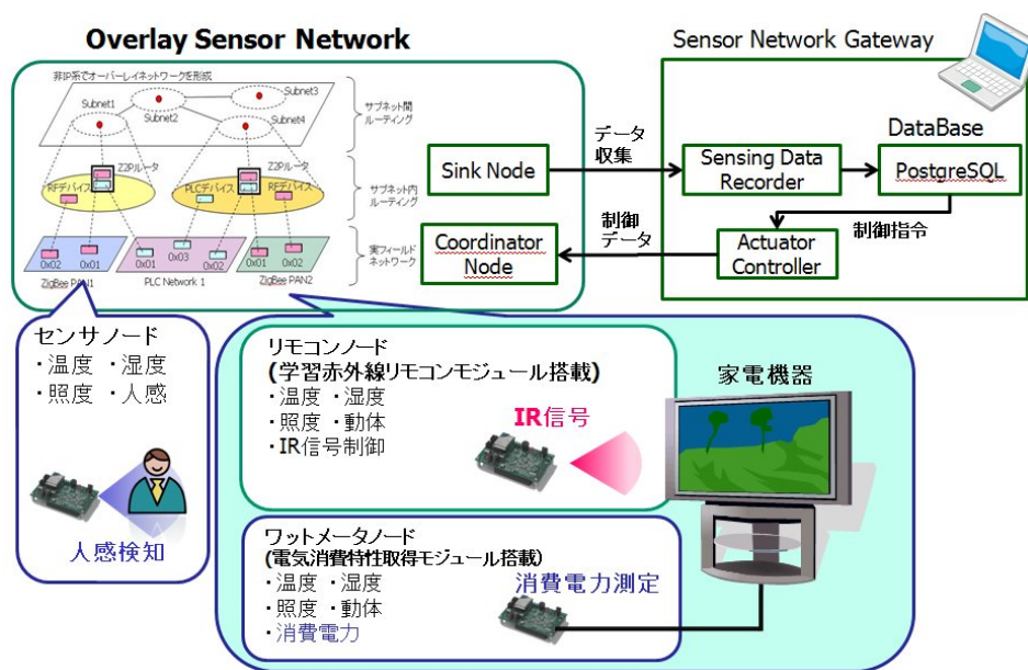
図3 PLC/ZigBee 相互補完通信を用いた省エネ制御システムのイメージ図
