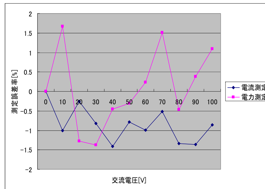
図8 白熱電球を負荷とした場合の電気消費特性取得モジュールの測定誤差 (0.5 級電気指示計器を基準としたグラフ)
