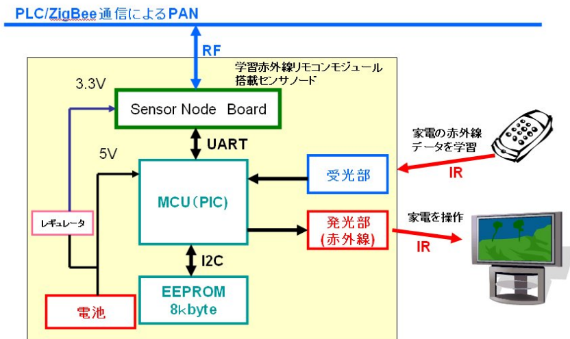
図7 学習赤外線リモコンモジュール搭載センサノードの概要図
