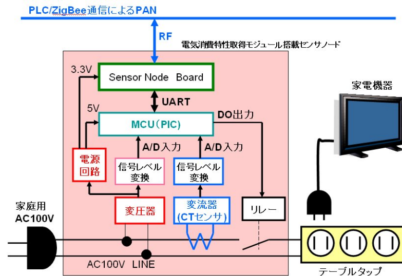
図6 電気消費特性取得モジュール搭載センサノード概要図
