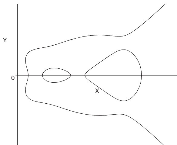
図-2 C_{45} 曲線の例
