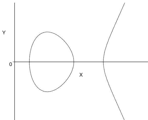
図-1 楕円曲線の例
