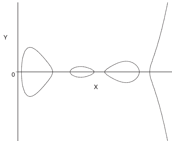
図-3 種数3の超楕円曲線の例
