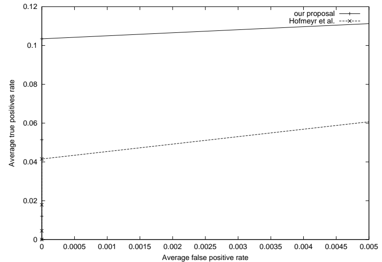
図6 psに関するデータを用いた異常検知の結果 (ROC 曲線) ( N = 6, D = 5 ) Fig. 6 The experimental result (ROC curve) using ps data set ( N = 6, D = 5 )
