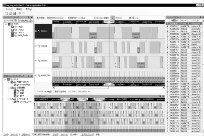
図 11 TOPPERS/FMP カーネルが出力するトレースログを可視化表示した TLV の実行結果のスクリーンショット
