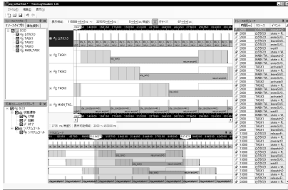
図 10 TOPPERS/ASP カーネルが出力するトレースログを可視化表示した TLV の実行結果のスクリーンショット
