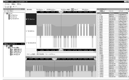
図 12 TECS のトレースログを可視化表示した TLV の実行結果のスクリーンショット
