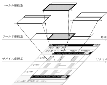
図 4 抽象的な可視化表示の仕組みの例
