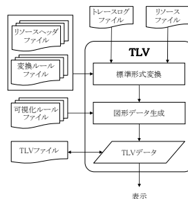
図 5 TLV の構成
