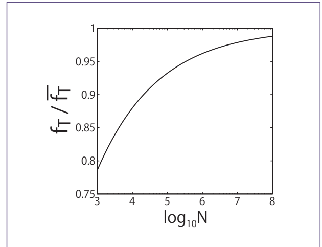
図-8 平均次数 \langle k \rangle = 3 のときの二極次数分布ネットワークの総ノード数 N に対する f_T / \bar{f}_T の振舞い。 N = 1000 ぐらいから約80%の強度を示し、 N = 10000 を超えると90%以上の強度を示す。
