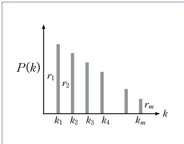
図-9 多極次数分布 (multimodal distribution). モード数 m を無限大にする極限でスケール・フリー・ネットワークの次数分布となる。
