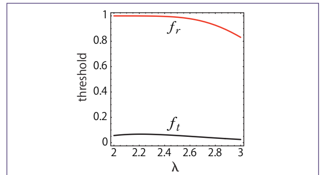
図-5 指数 \lambda を持つスケール・フリー・ネットワークのノード除去閾値。広い範囲で f_r \approx 1 である一方で f_t は10%にも満たない。
