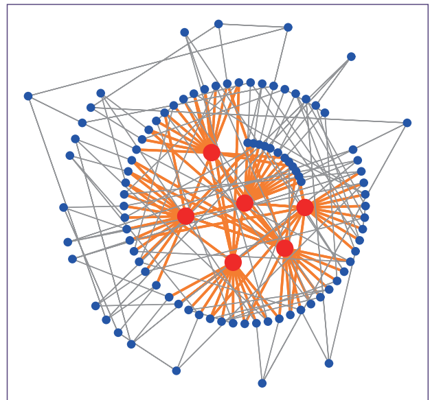
図-10 総ノード数 N=100 、平均次数 \langle k \rangle \approx 3 の場合に最適化された二極分布ネットワーク. この場合、必要なハブ (赤いノード) は 6 つであり、その次数は 17 である. その他の 94 個のノード (青) は平均次数 3 を持つ.
