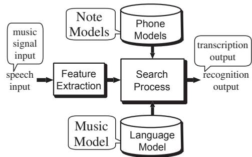
図-6 連続音声認識システムの自動採譜への転用
