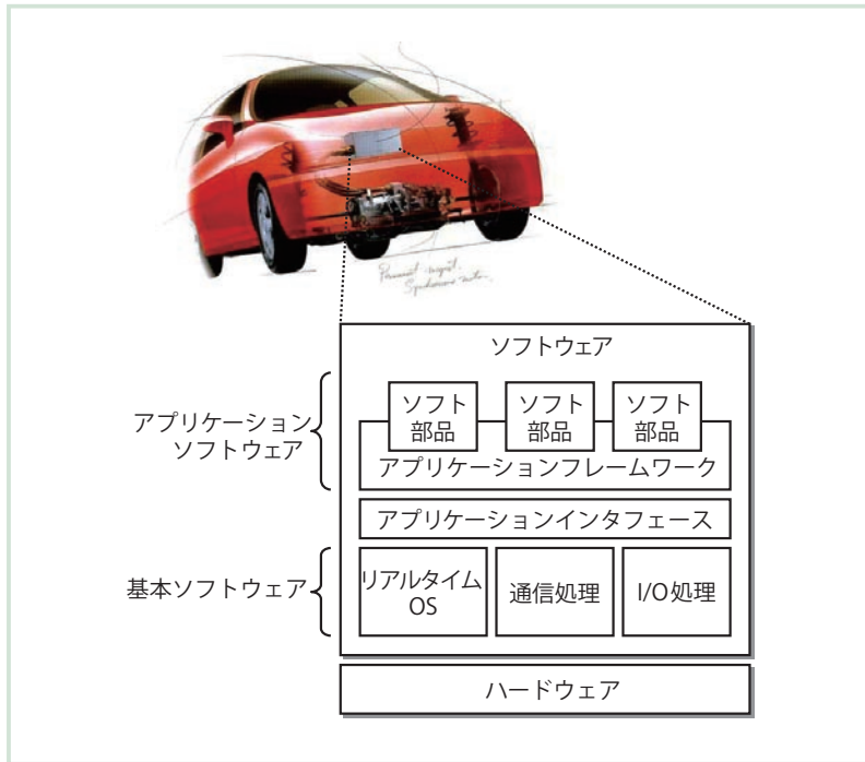
図-2 自動車向け組み込みソフトウェア
