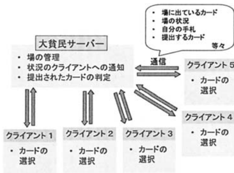
図 2: システム構成図 (1)
