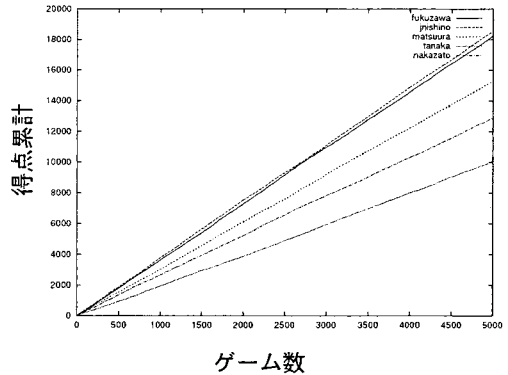
図 9: 決勝戦結果 得点推移
