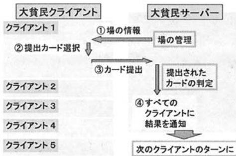
図 3: システム構成図 (2)
