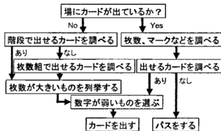
図 4: 提出カード選択のフローチャート
