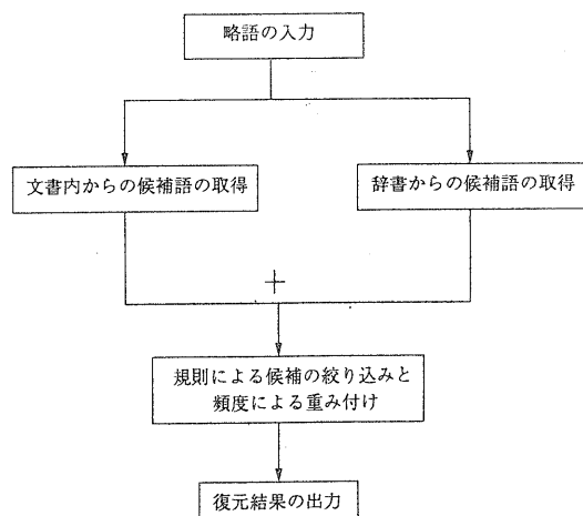
図1: 略語復元処理の流れ
