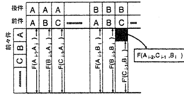
図 6: 選択的 tri-gram
