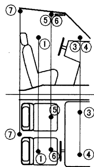
図 1 マイクロホンの設置位置（上段）：側面，（下段）：真上 Fig.1 Microphone positions for data collection: Side view (top) and top view (bottom).
