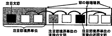
図4 節境界単位で閉じていない係り受けの係り文節の検出において着目した言語単位
