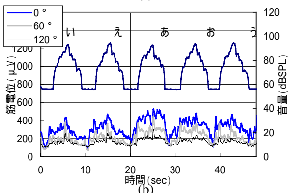
図 13 : モード 3 (被験者 A, 音量と筋電位, ピッチ)
