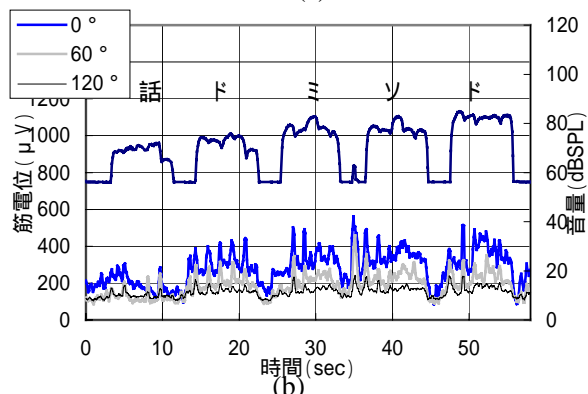
図 16 : モード 4 (被験者 A, 音量と筋電位, ピッチ)
