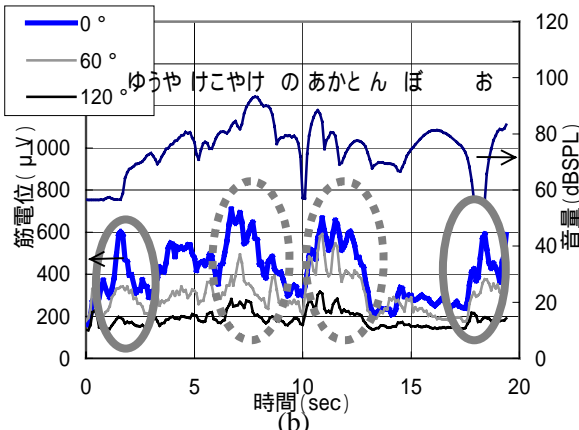
図4：音量と筋電位及びピッチ（被験者A）
