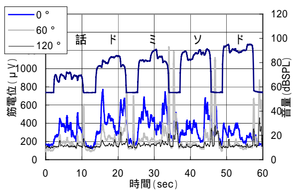
図 18 : モード 4 (被験者 C, 音量と筋電位)
