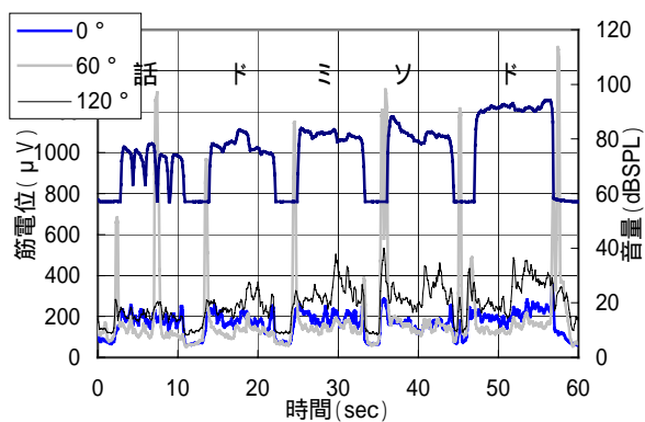
図 17 : モード 4 (被験者 B, 音量と筋電位)
