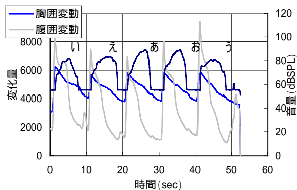
図21：モード2（被験者C，音量と呼吸情報）
