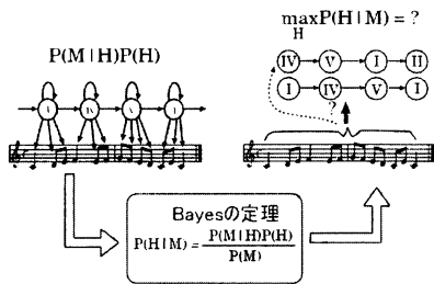
図 2: 旋律生成モデルと和声付け問題の対応 [7]
