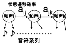
図 3: 2 和声間遷移モデル
