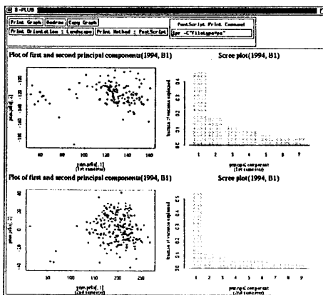
図 8: 主成分分析
