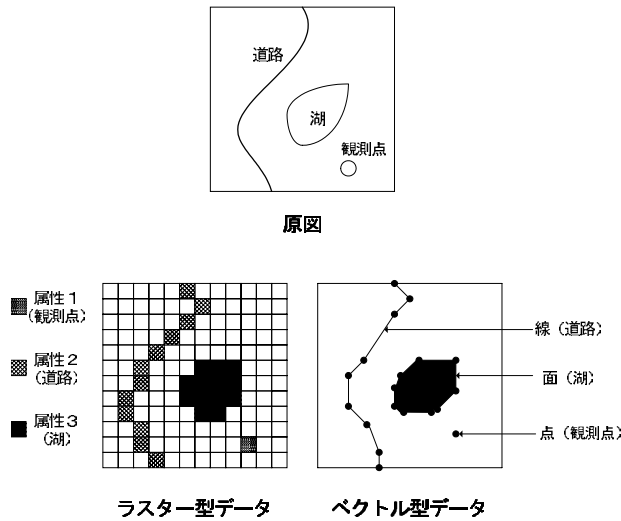
図 2: それぞれのデータ構造
