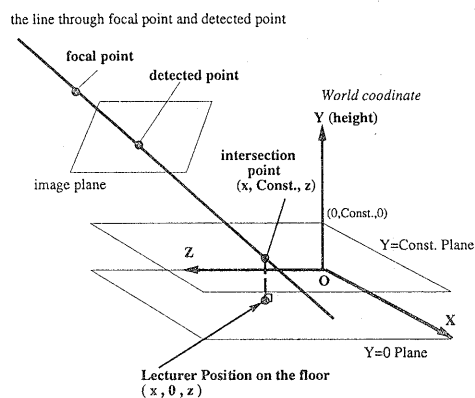
図 2: 単眼カメラによる講師位置の検出
