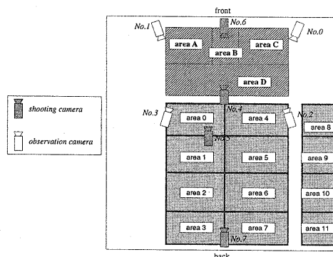
図1: 京都大学附属図書館 AV ホールにおける領域分割
