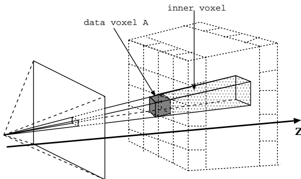
図 6 距離データ点によるボクセル空間への投票 Fig. 6 Voxel voting.
