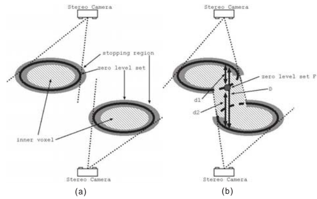
図 7 停止領域と内部ボクセル Fig. 7 stopping region and inner voxel.
