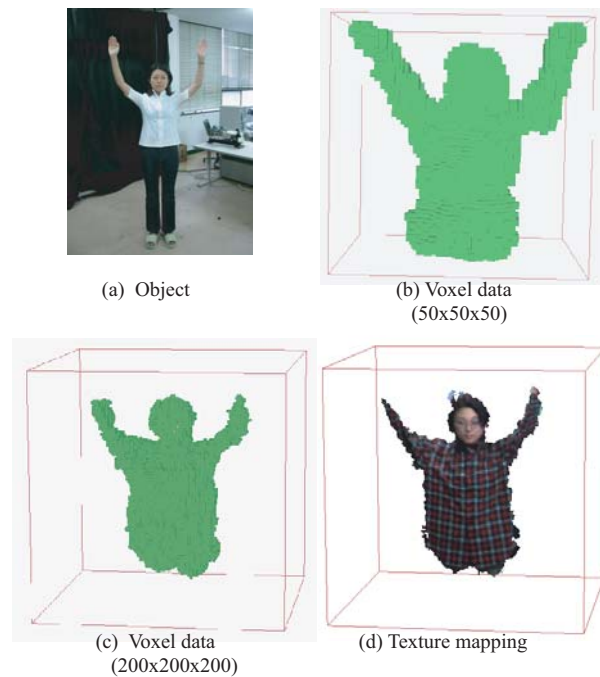
図 8 3 次元人体形状の復元 Fig. 8 3D reconstruction of human body.
