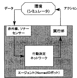
図1 エージェントの構成
