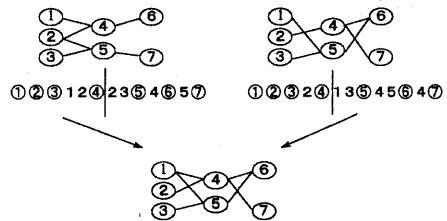
図2 ネットワークの表現型と染色体表現及び交叉の例
