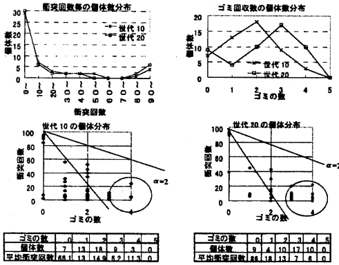
図 13 10 世代と 20 世代の個体分布
