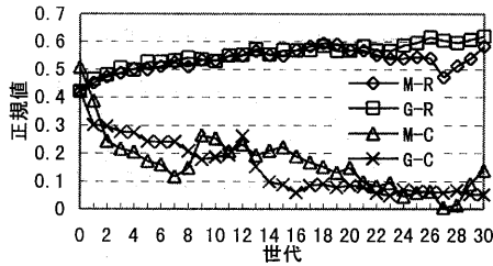
図6 拡張多目的GA(M)と単純なGA(G)の進化の比較
