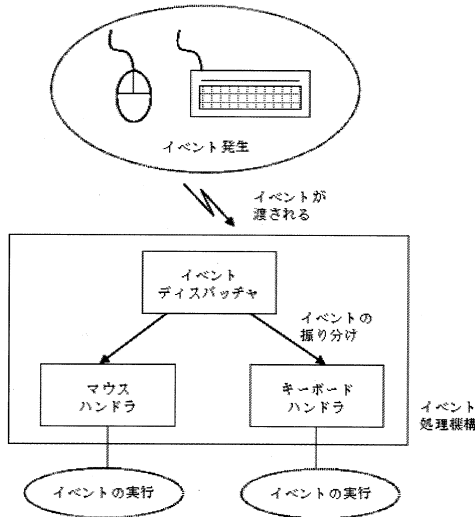
図3 GUI方式のイベント処理機構の概念 Fig.3 Event driven model of a GUI
