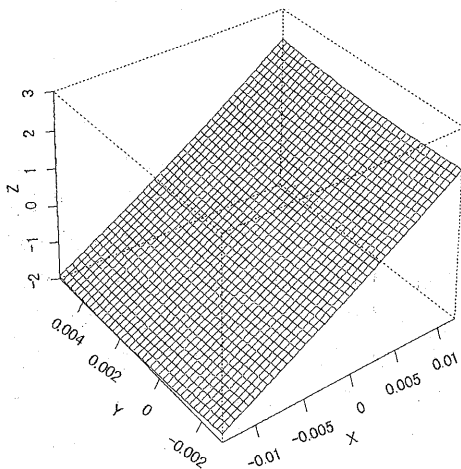
図 3：関心モデル
