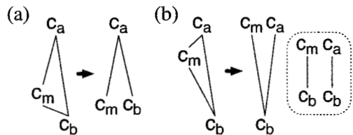
図 2: オントロジーの構造の修正
