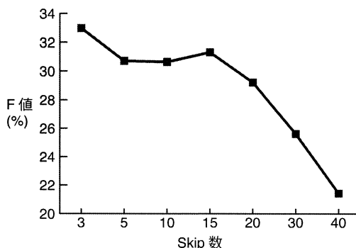
図 4: skip 数による F 値の変化
