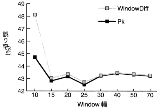
図 1: 雑談コーパスにおける DiaSeg の性能
