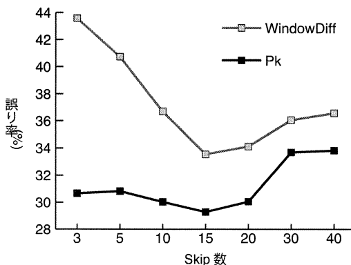
図 3: skip 数による Pk 及び WindowDiff の変化
