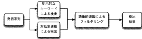
図 2: 提案手法の流れ
