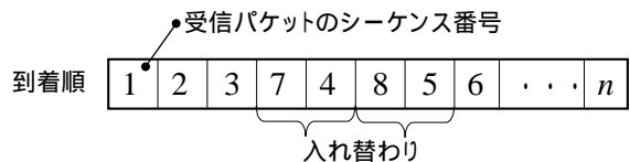
図3. パケット順序エラーの導出
