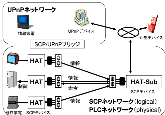
図 1 システム外観
