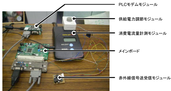
図 4 HAT プロトタイプ外観
