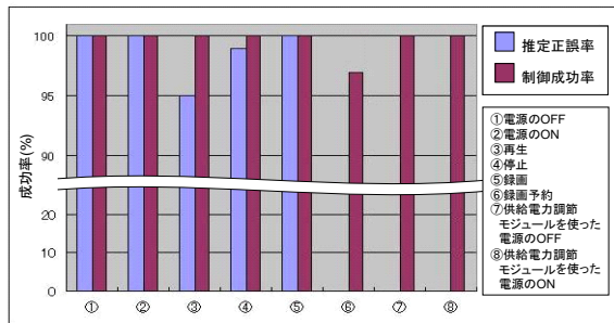
図9 プロトタイプ評価実験結果
