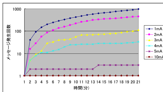
図 5 変動幅とメッセージ発生回数の相関図
