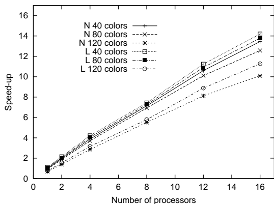
図 4 有限要素解析ベンチマークにおける速度向上 (N: ノーマルページ使用, L: ラージページ使用) Fig. 4 Speed-up in finite element analysis benchmark (N: normal page case, L: large page case)
