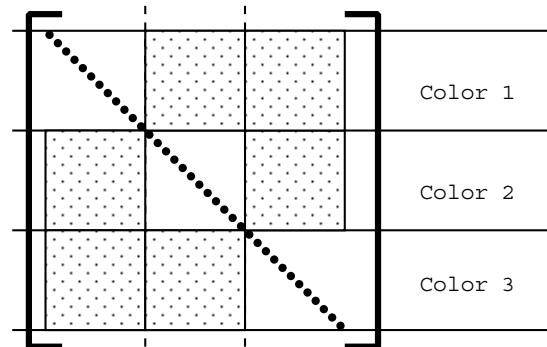
図1 マルチカラーオーダリング法における係数行列 Fig. 1 Coefficient matrix in multi-color ordering method
