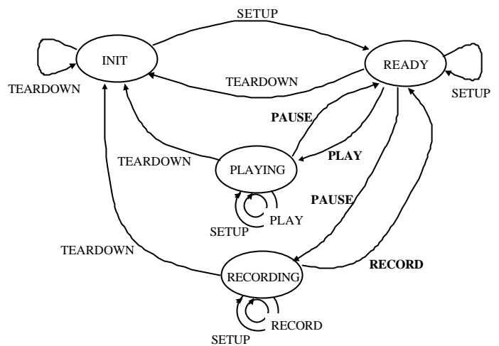
図 3：mRTSP/RTSP 状態遷移図
