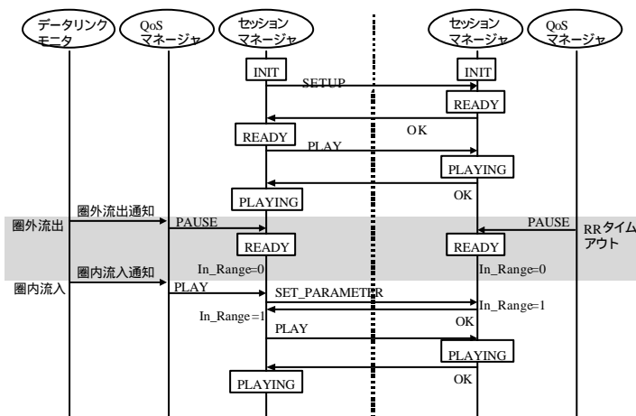
図5：圏外流出時（短時間）のシーケンス
