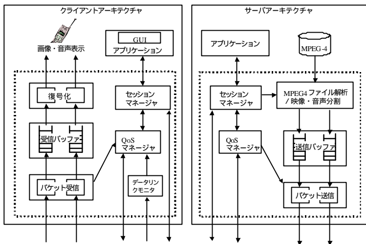
図 8 : モバイル QoS システム構成図
