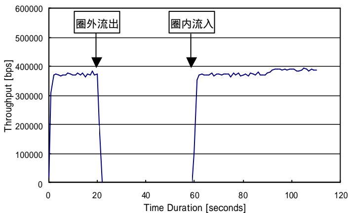
図9：圏外・在圏試験時のスループット時間変化
