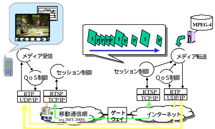
図1：マルチメディアストリーミングシステム全体図
