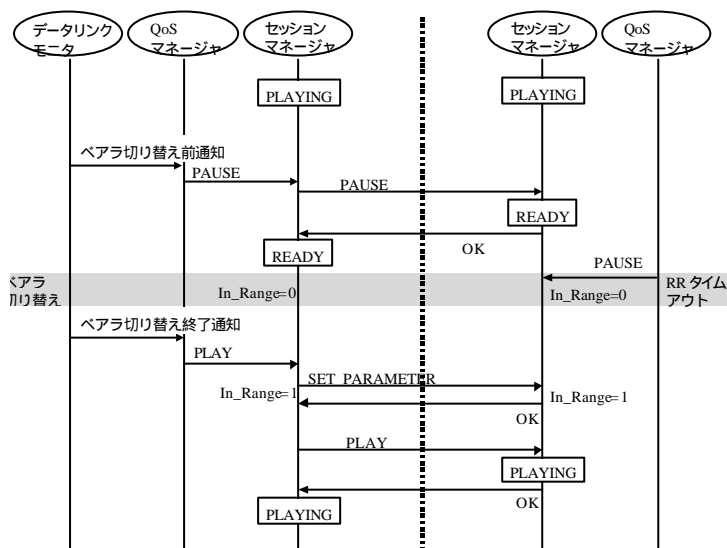
図 7 : ペアラ切り替え (IMT-2000/無線 LAN) 時のシーケンス
