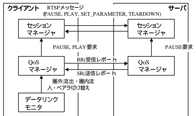
図 2：セッション制御主体構成図
