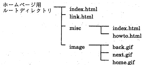
図 2(a): ホームページデータの木構造
