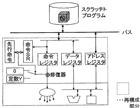
図6: スクラッチ方式として再構成されたCPU
