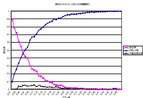
図5. 2相コミットメントシミュレーション結果 (時間差あり)
