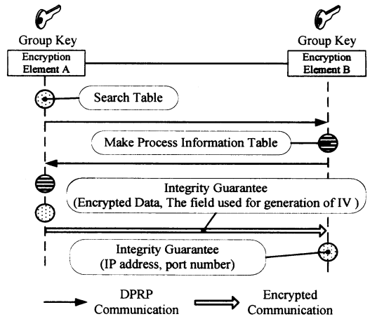
図 9 DPRP と組み合わせたパケットの完全性保証 Fig. 9 Packet Integrity combined with DPRP.
