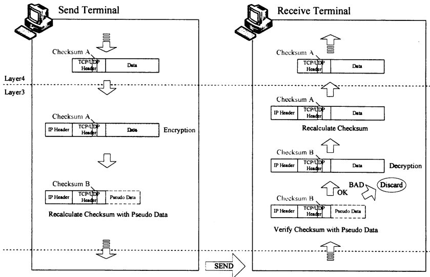
図 8 チェックサムの演算方法 (End-to-End の場合) Fig. 8 Flow of the Checksum execution (case of End-to-End).
