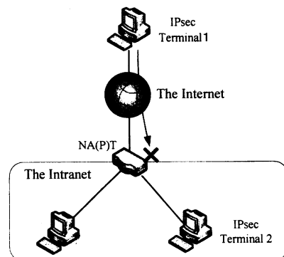
図 1 トランスポートモードで NA(P)T を経由する例 Fig.1 Example of NA(P)T traversal with transport mode.
