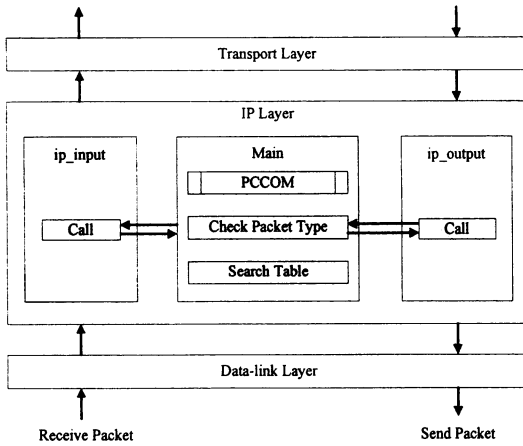
図 10 試作システムの実装方式 Fig.10 Implementation of the trial system.
