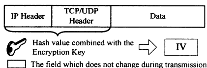
図 6 IV (Initialization Vector) の生成
