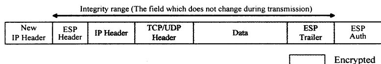
図 3 ESP トンネルモードの packets フォーマット
