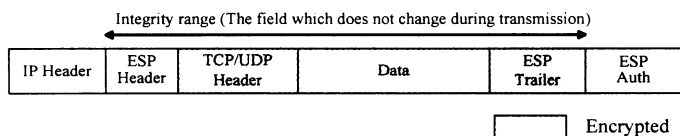
図 2 ESP トランスポートモードの packets フォーマット
