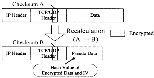
図 7 疑似データによるチェックサムの再計算 Fig. 7 Recalculation of Checksum with Pseudo Data.
