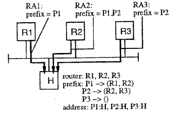
図 6 ネットワーク構成例
