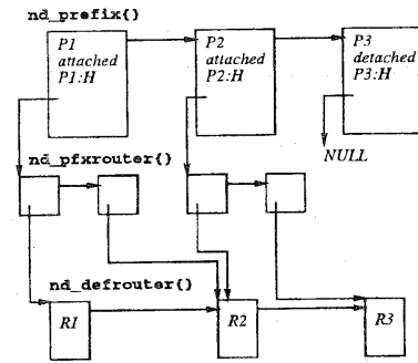
図 7 カーネル内のデータ構造
