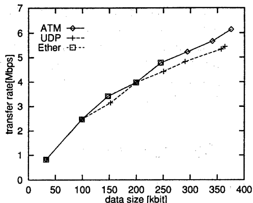
図4: ネットワークスループット (ビデオボードを使用した場合)
