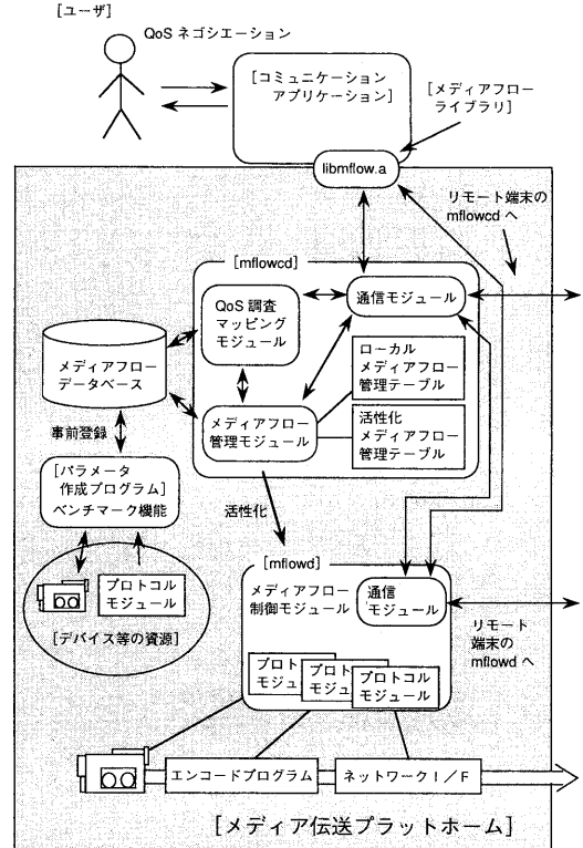
図 3: メディア伝送プラットフォームの実装
