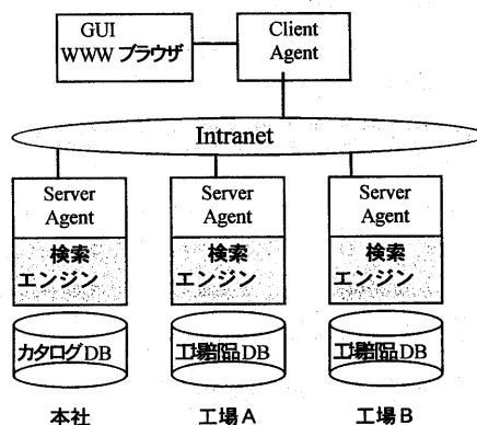
図4. 1 開発した検索エージェントの構成（検索エンジンの書き換えのみで新しいDBが追加できる）
