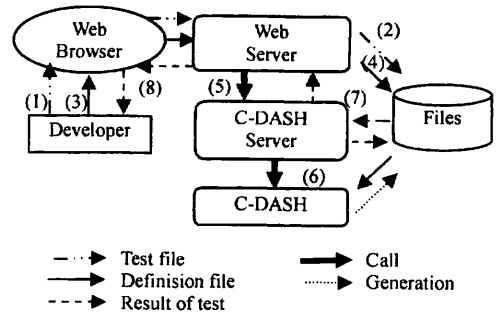
図 3 テストファースト開発の流れ
