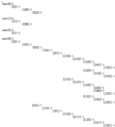
図 8: アルゴリズム 1 を図 7 の (a) に適応した結果リスト構造の例
