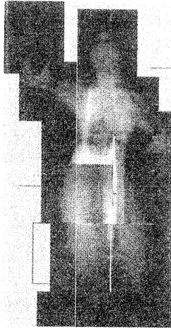
図 1: 仏像の X 線写真(図 2,3 とは異なる仏像)
