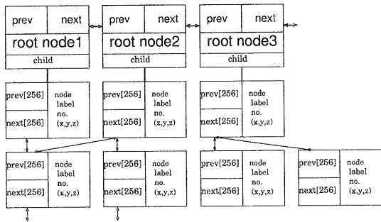
図 4: データ構造
