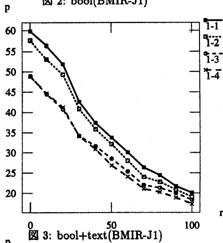
図 2: bool(BMIR-J1)
