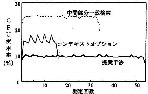
図5： 評価実験1の結果（CPU使用率）
