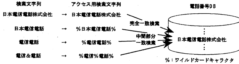
図1： 電話番号検索の例
