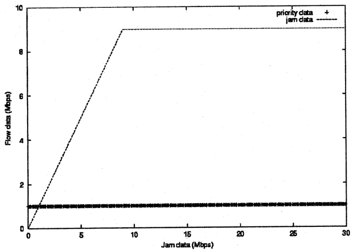
図 3. メタデータによる優先制御を行った通信
