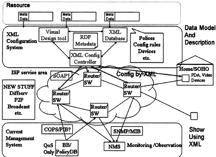
図 1. メタデータによるネットワーク制御のアーキテクチャ
