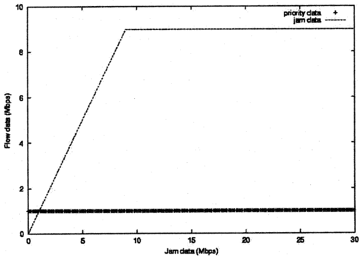
図2. メタデータによる優先制御を行わない通信
