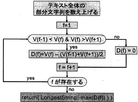
図3 検出の流れ
