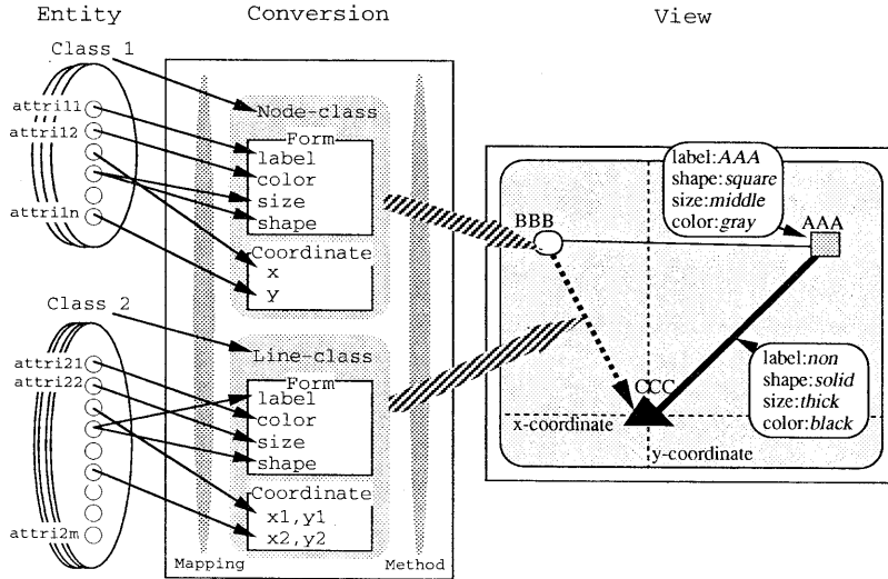
図3 ノードラインビューモデルの実装例
