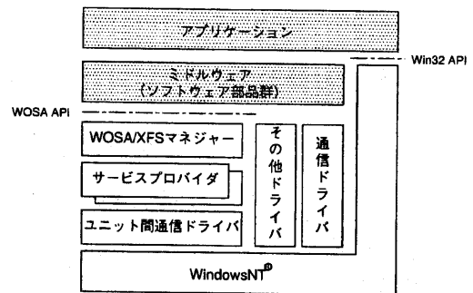
図 1: CW-500 のソフトウェア構造
