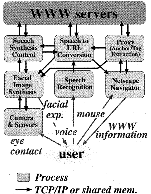
図 3: VPA implementation
