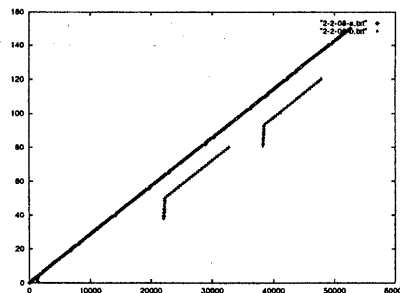
図 4-2: イベント型同期 (コネクション 2, バッファサイズ=8)
