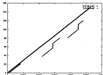
図 4-3: 部分型同期 (コネクション 2, バッファサイズ=8)
