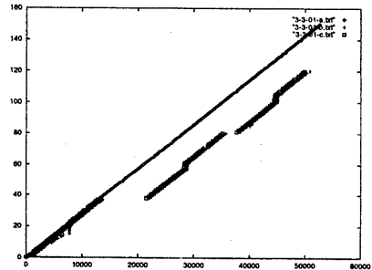
図 4-7: 部分型同期 (コネクション3, バッファサイズ=1)
