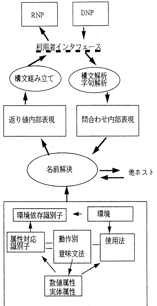
図 2: 記述名 名前管理の全体図
