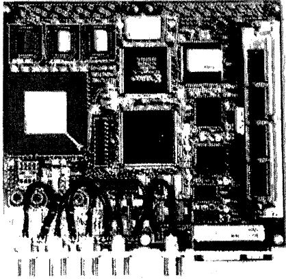
図2 IPパケットの監視ボード
