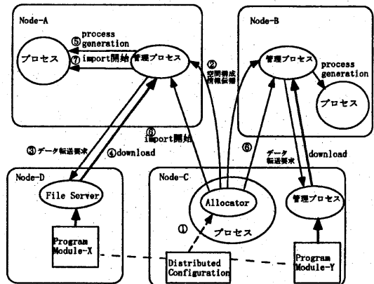
図9. Allocatorと管理プロセス
