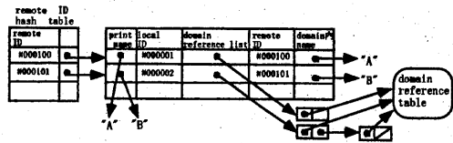
図4. Local Reference Table
