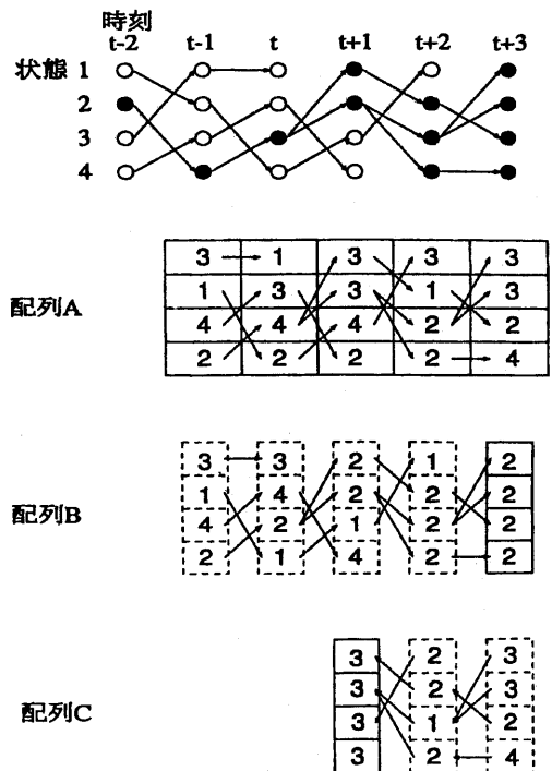
図3 ロザリオ型パス探索法において使用する配列
