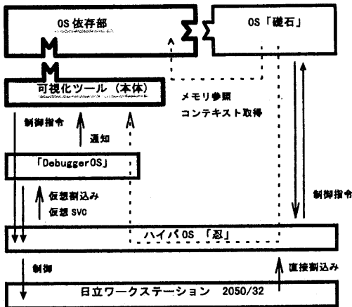
図 6.2 全体構成
